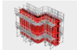
FRWF Coffrage De Voiles Avec Peau Coffrante Acier
