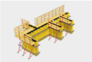
H20P Coffrage De Voile Avec Peau Coffrante En Contreplaqué
